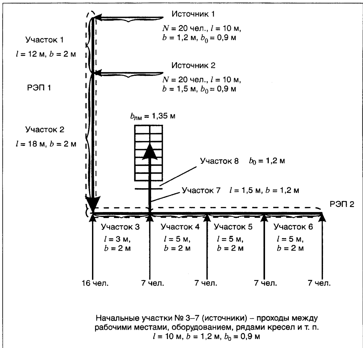
Рис. П5.2. Пример составления расчетной схемы эвакуации людей по части этажа до входа в лестничную клетку: N – количество людей; b – ширина; l – длина; b_0 – ширина проема 0
