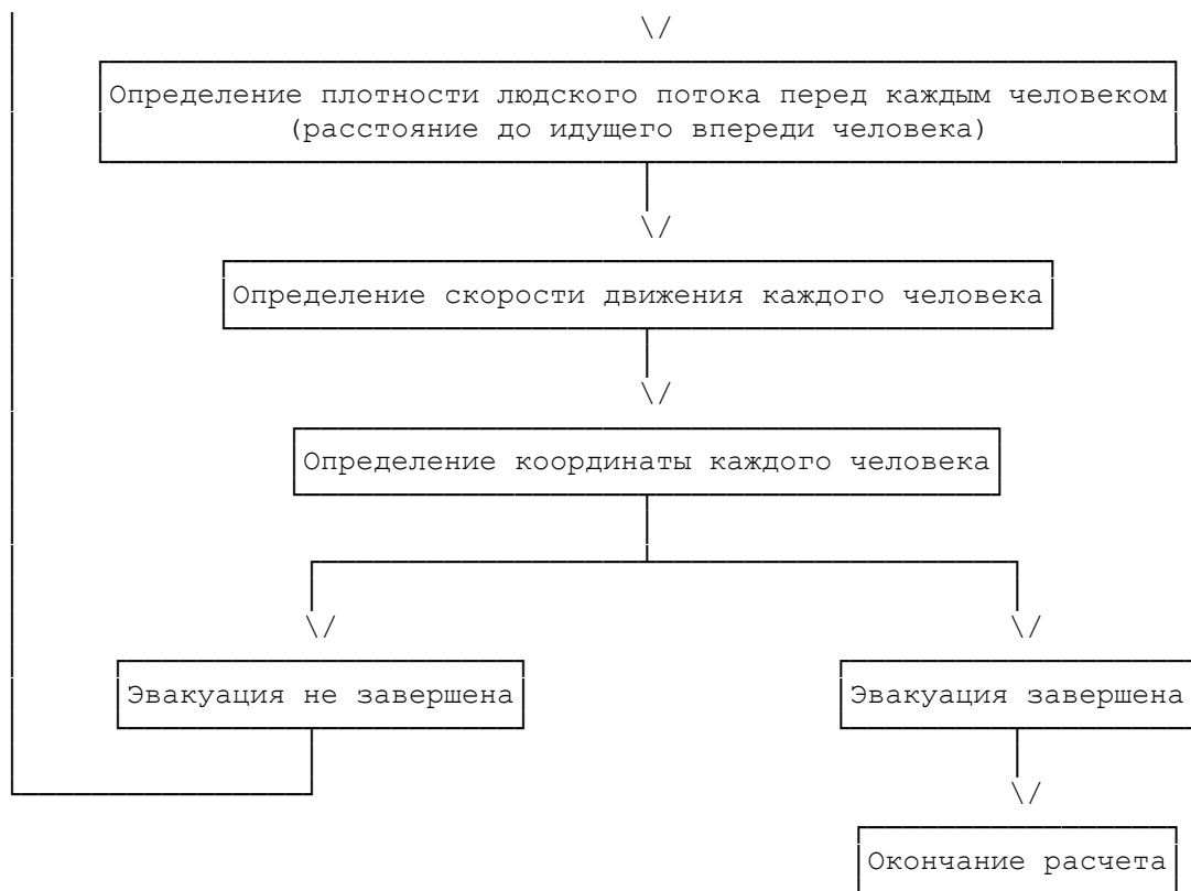
Рис. ПЗ.2. Блок-схема определения расчетного времени эвакуации людей из здания
