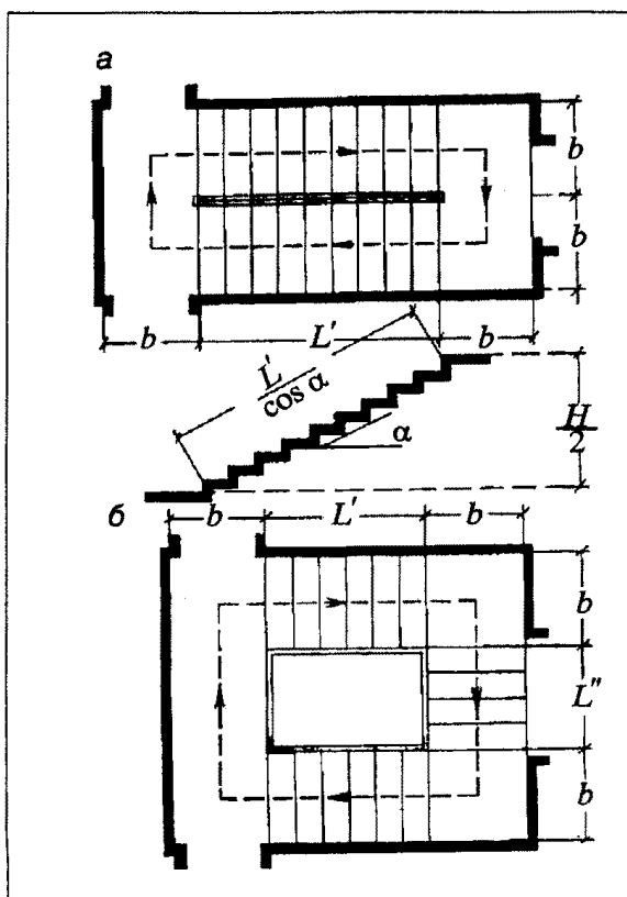
Рис. П5.1. Расчетная длина пути по лестнице: а - двухмаршевая лестница; б - трехмаршевая лестница
