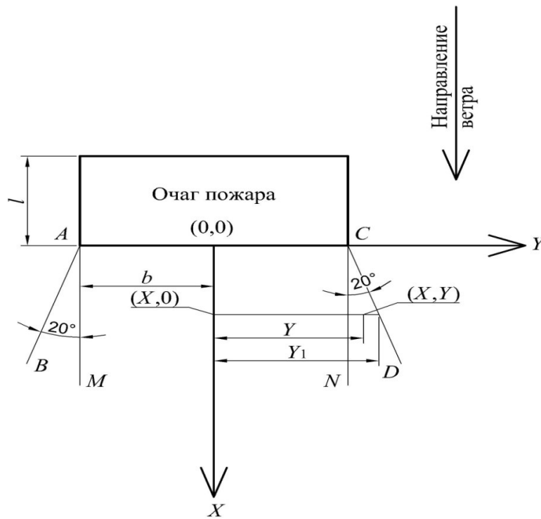
Рисунок E.1 – Схема определения размеров зон загазованности от отдельного очага при направлении ветра перпендикулярно к фасаду здания
