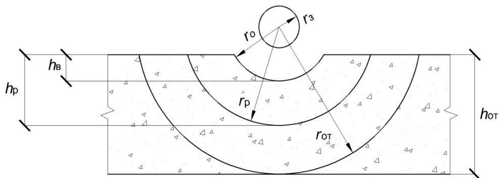
Рисунок Б.2 – Области разрушения преграды при взрыве
