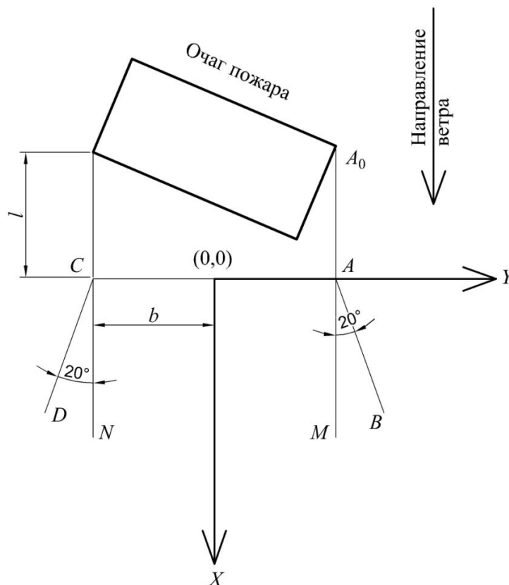
Рисунок E.2 – Схема определения размеров зон загазованности от отдельного очага пожара при направлении ветра под острым углом к фасаду здания
