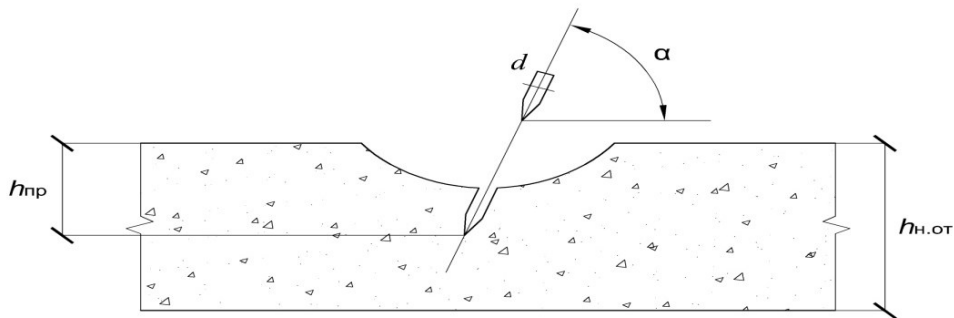
Рисунок Б.1 – Области разрушения преграды при ударе
